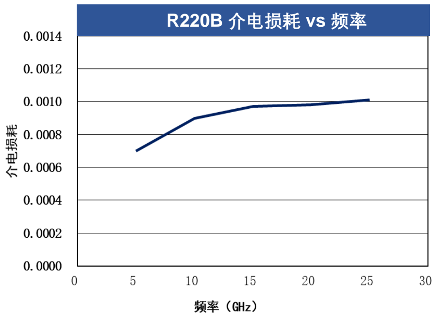
图 2 证明了损耗随频率变化的稳定性。 这个特性证明了睿龙 R220B 跨频率的固有稳定性，为高频应用中信号完整性作为整体性能关键性部分提供了一个稳定的平台。
