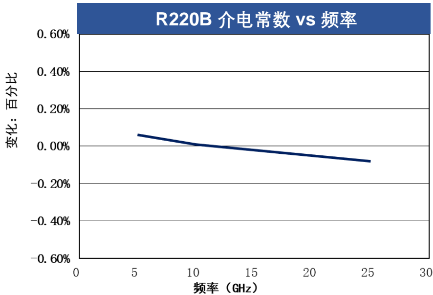
图 1 证明了介电常数随频率变化的稳定性。 这个特性证明了睿龙 R220B 跨频率的固有稳定性，从而可简化整个电磁频谱范围的设计，R220B 介电常数在整个频率范围的稳定性确保设计及放大的稳定性。
